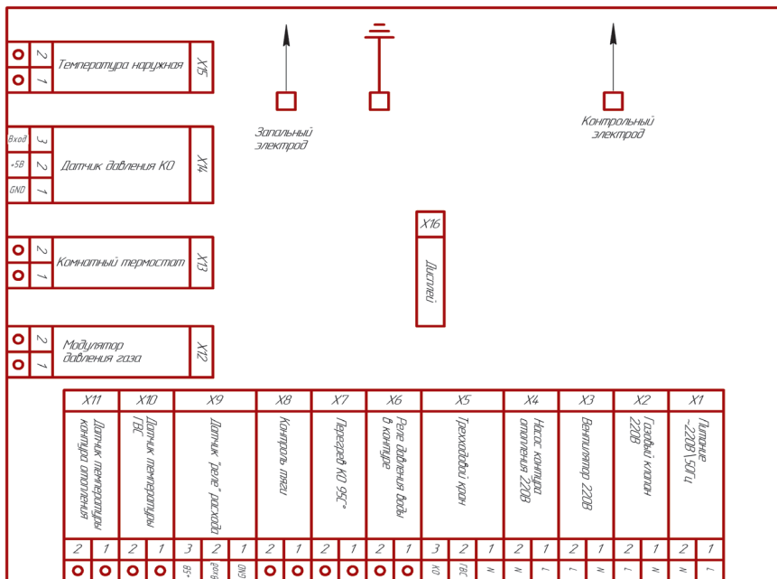
Рис. 9. Подключение дополнительных устройств
